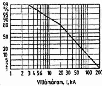
11. ábra A villámáram-csúcsérték ( I ) értékeinek gyakorisága
