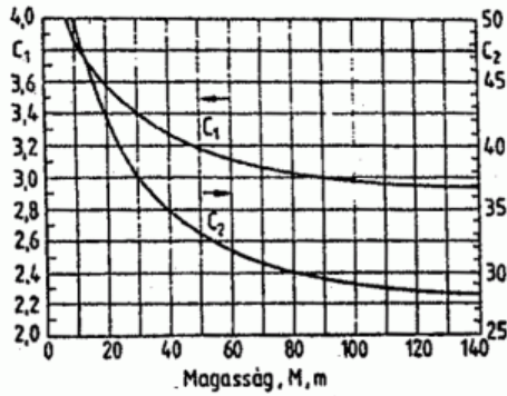
9. ábra A C 1 és C 2 együtthatók értékei az M építménymagasság függvényében
