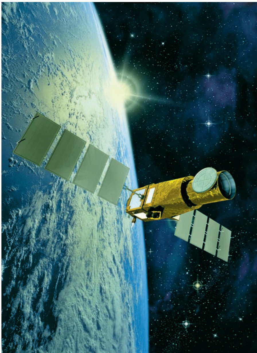
A COROT-űrszonda
