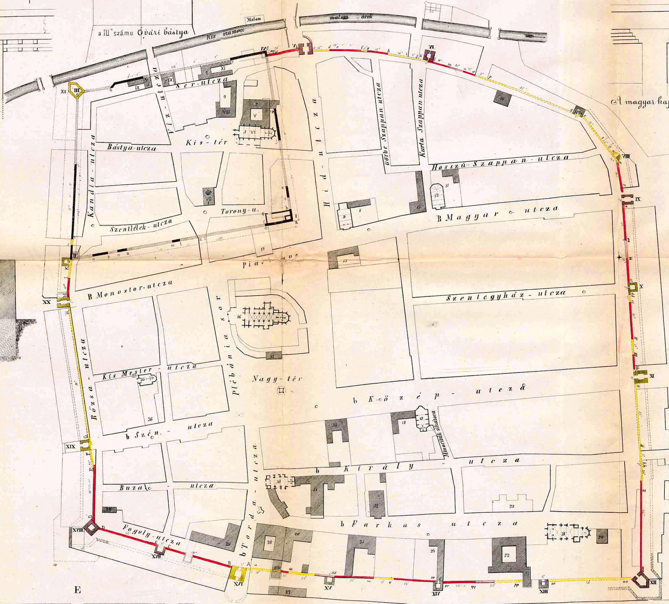
E a Bethlen bástya melletti várfal rész
