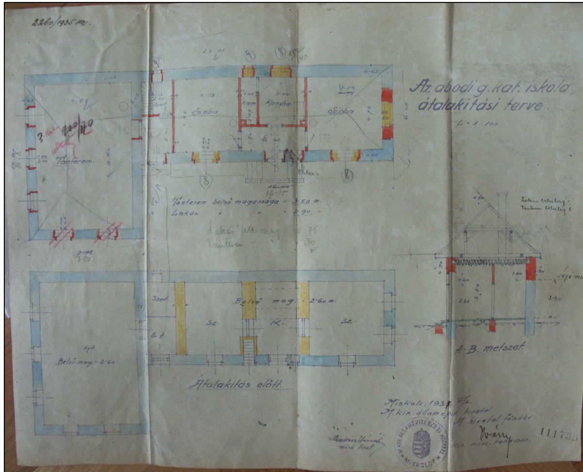
Az iskola átalakítási terve. (A szerző felvétele)
