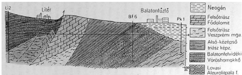
Földtani szelvény Litér és Balatonfűzfő között [1]
