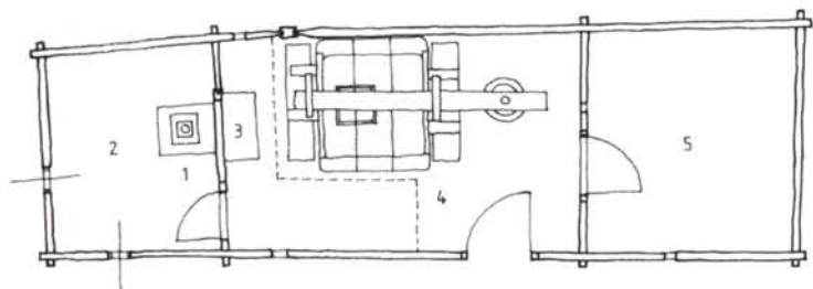
59. Háromhelyiségű présház alaprajza: 1. Szoba kívülfűtős cserépkályhával; 2. Présház tüzelő padkával, préssel; 3. Pince.
