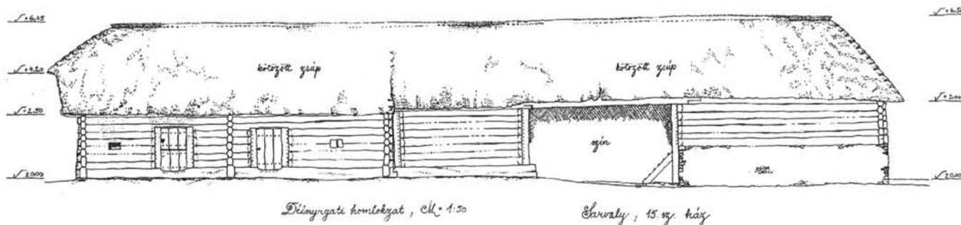
81. Füstösház Sarvalyon (15. sz. ház). Rekonstrukció.
