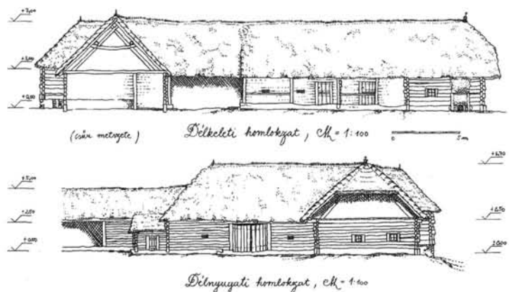
Sarvaly, 17. gómi lakóház rekonstrukciós terve
