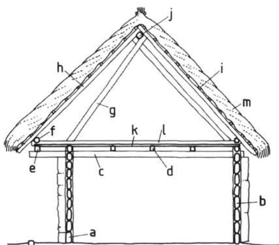
29. A boronaház részei: a) talpborona, b) falborona, c) mestergerenda, d) födémgerenda, e) koszorúgerenda, f) talpszelemen, g) ollószár, h) szarufa vagy „rag”, i) tetőléc, j) szelemen, k) födémdeszka, l) tapasztás, m) zsúptető
