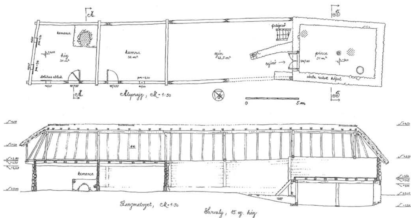
82. Füstőház rekonstrukció. Felül: alaprajz, alul: metszet. Sarvally (15. sz. ház).
