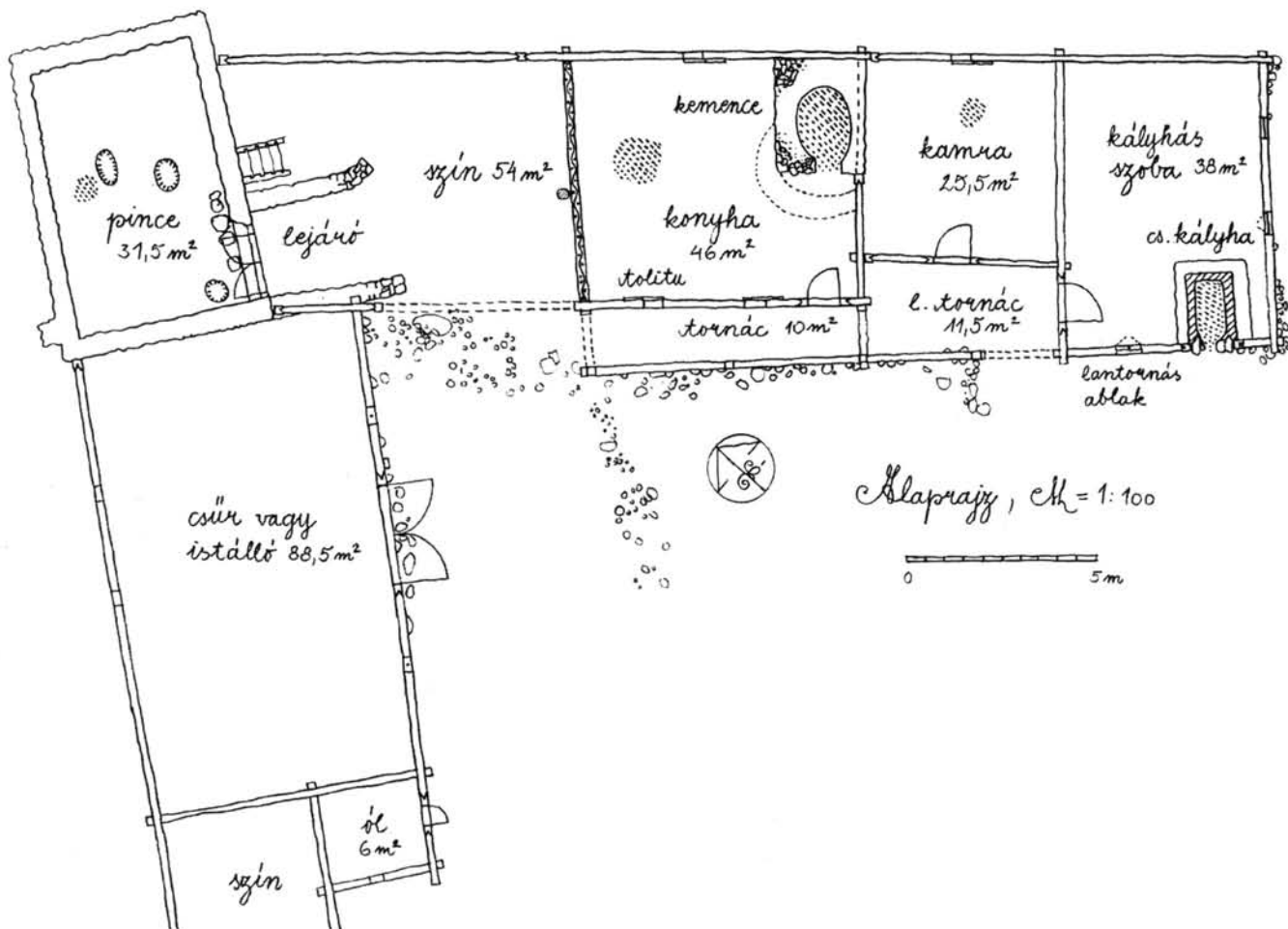
83. Kályhás szobás ház Sarvalyon (17. sz. ház).
