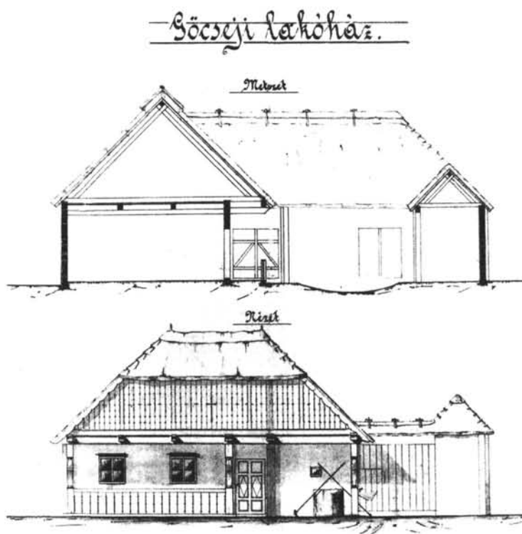
101. Kerített lakóház udvari homlokzata bodonkúttal, Lenti, 1893.
