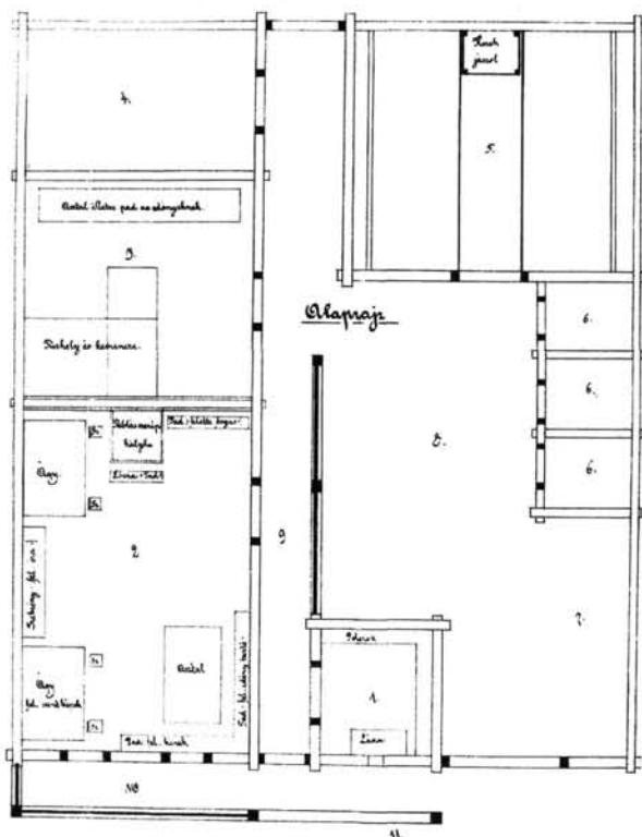
102. Az előző lakóház alaprajza. A rajzon jól látható a szobai bútorok elrendezése.
