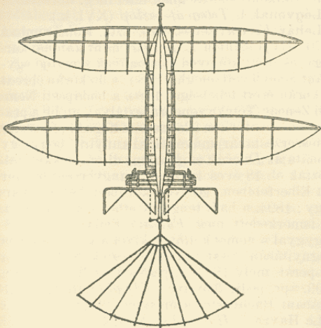
2. ábra. Kress repülőgépe.
