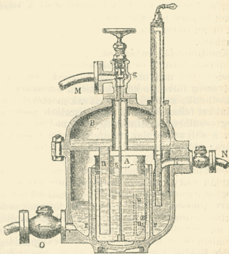
Schauer-féle levezető készülék.
