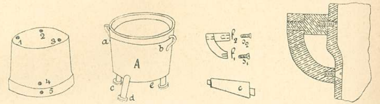
15—18. ábra. Vasfazék sárgarézből készített mintája.
