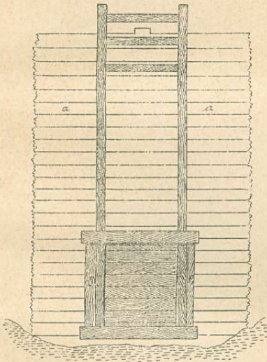
5. ábra. Létrás szerkezetű tiltókészülék, a) vízfal, b) tiltóvezeték.
