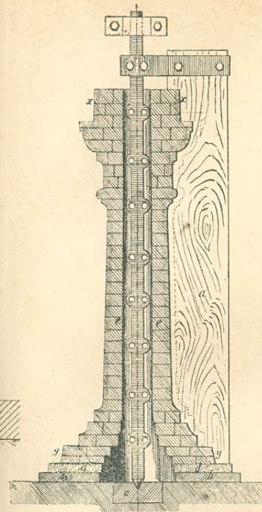
32. ábra. Oszlop beformázása alkzóval.
