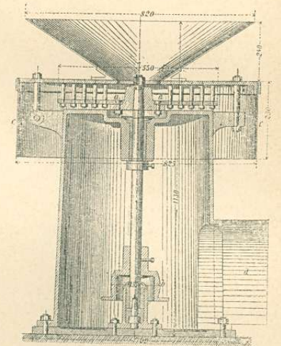
6. ábra. Vasgyűjtővel felszerelt kupolókemence.
