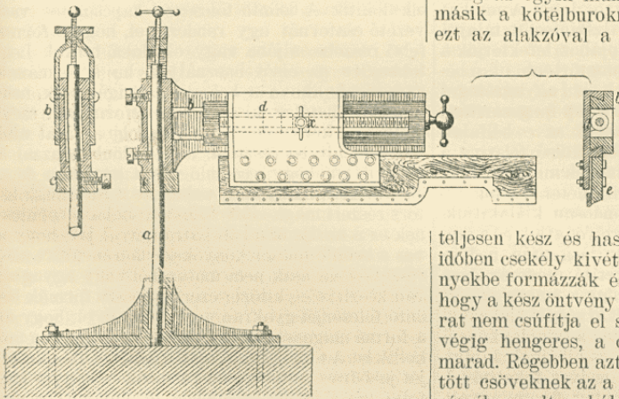
27–28. ábra. Az alakzó (sablon) elrendezése.
