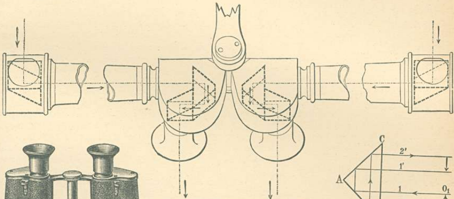
7. ábra. A prizmák elrendezése és a sugár útja a relief-távesőben. Vázlatosan.
