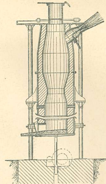
7. ábra. Herbertz-féle kupolókemence.
