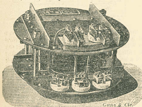
5. ábra. Ganz és társa transzformátora.
