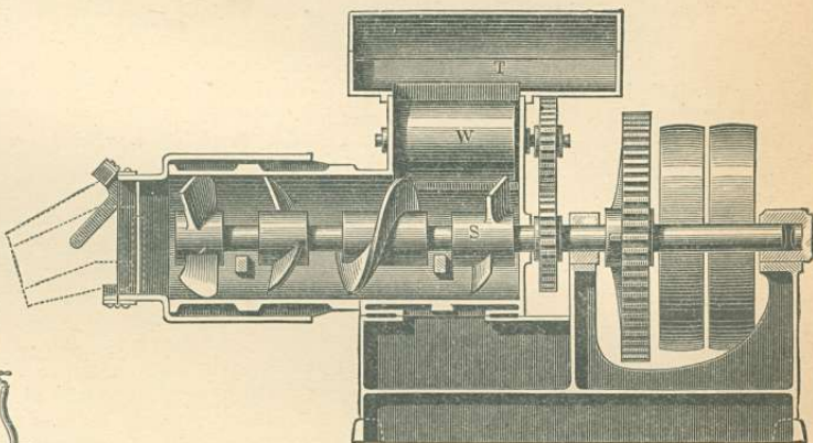
4. ábra. Schlickeysen-féle tőzeg gép gőzerőre.
