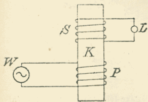
1. ábra. Váltóáram-átalakító.
