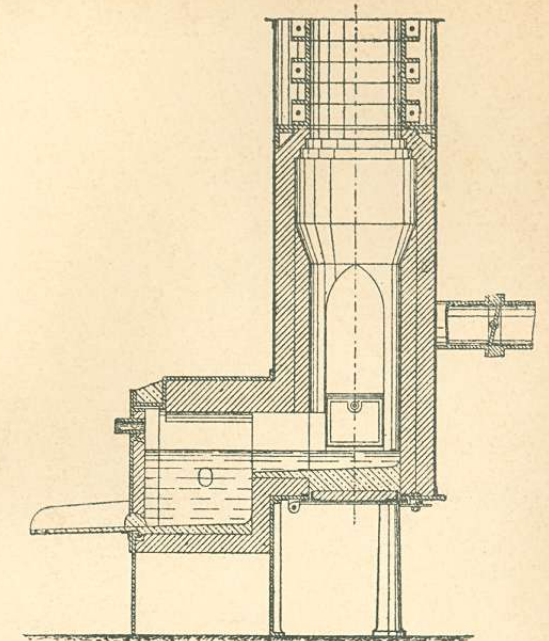
6. ábra. Vasgyűjtővel felszerelt kupolókemence.
