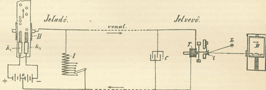
2. ábra. A gyorstelegráf általános elrendezése.
