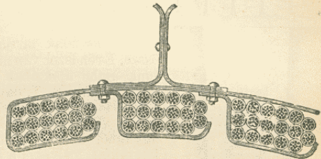
1. ábra. Vasbádó-gtartószerkezet.
