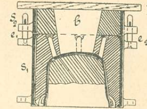
19—22. ábra. Vasfazék befornázása.
