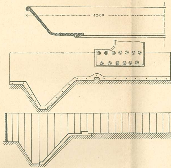
29—31. ábra. Körkerek gépágy befornázása.
