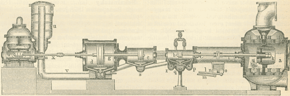
1. ábra. Worthington-féle háromszorosan expandáló gőszivattyú hosszmetzete.
