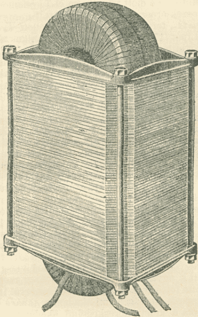
8. ábra. Westinghouse Company köpeny-transzformátora.
