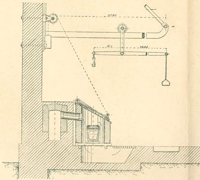
10. ábra. Tégelykemma.
