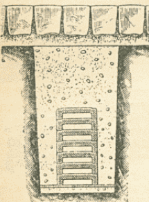
5. ábra. Kábelcsatorna több emeletre, cémentből.
