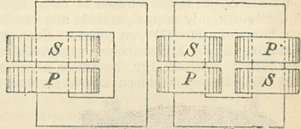
2—3. ábra. Vasmag-transzformátor.
