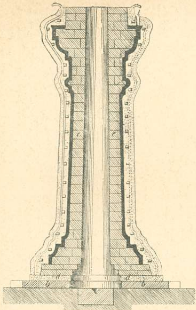
33. ábra. Oszlop befornázása alakzóval.
