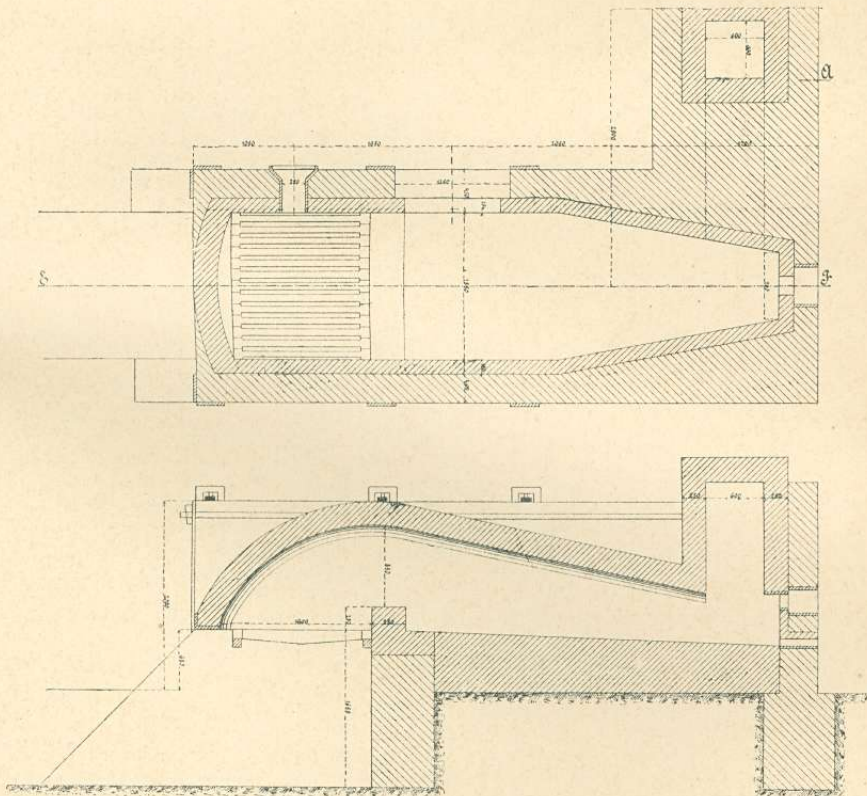
8—9. ábra. A lángálló alaprajza és hosszanti metszete.
