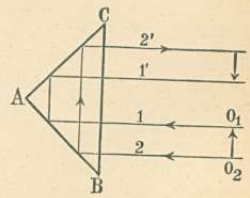
1. ábra. Teljes visszaverődésű prizma.
