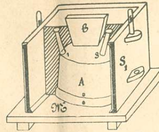
19—22. ábra. Vasfazék befornázása.
