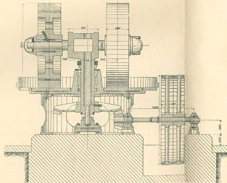
3. ábra. Agyaggyúrásra való korongpár alul elrendezett hajtószerkezettel.
