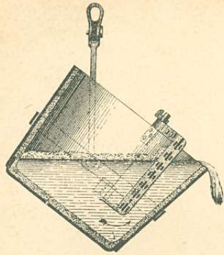
12. ábra. Öntőüst salakvisszatartó rekesszel.
