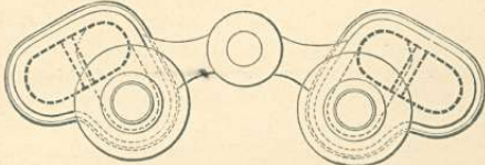
4. ábra. Kettős táveső fölülről nézve.
