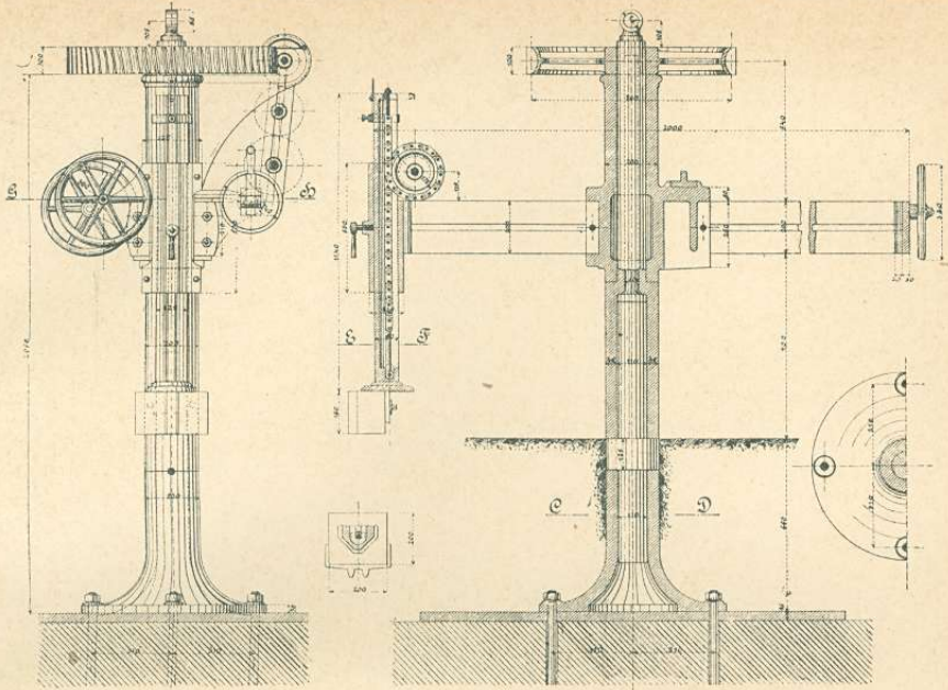
34—35. ábra. A formázógép előlnézete és hosszanti metszete.
