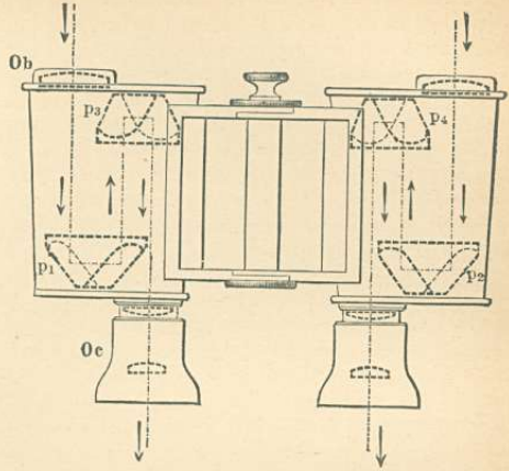
3. ábra. Kettős táveső hosszszelvénye. A prizmák elrendezésének s a sugár útjának vázlatos rajza.
