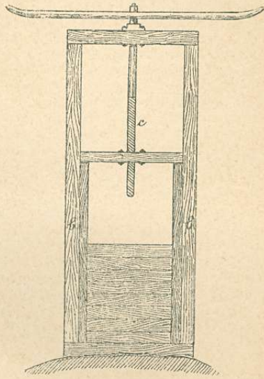
6. ábra. Csavaros szerkezetű tiltókészülék, b) tiltóvezeték, c) csavar.
