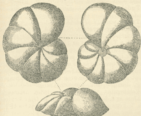
Truncatulina grosserugosa.
