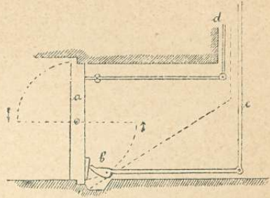
4. ábra (hosszmetszet). a) Vízszintes tengelyű csapókapu vasból, b) a csapókapu nyitására szolgáló o tengely körül forgó emeltű, c) a gát koronájáig érő lánc, d) a csapókapu bezárására szolgáló lánc.
