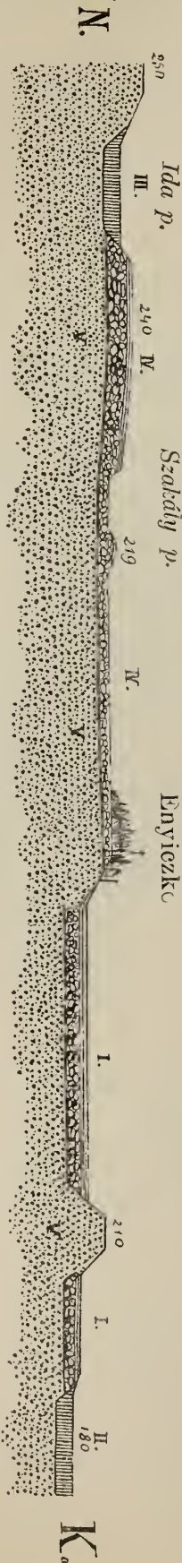
AZ ENYICZKEI FENSÍK ÁTMETSZETI KÉPE. I. A Hernád diluviális ártere. II. A Hernád jelenkori ártere. III. Az Ida patak jelenkori ártere. IV. Diluviális agyag, kavics és homok. V. Pontusi képződmények. Mérték a hosszúságra = 1 : 50,000. — Mérték a magasságra = 1 : 5,000.
