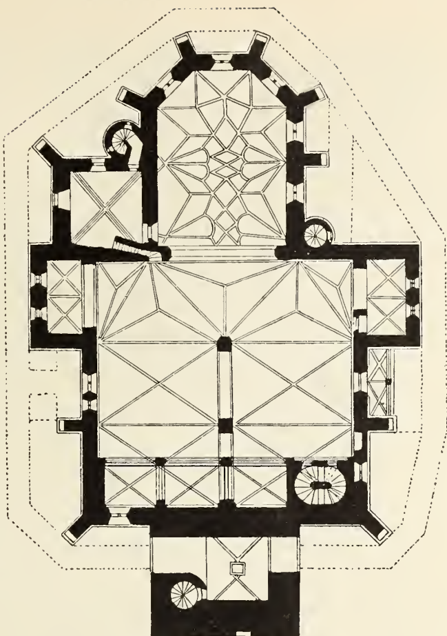
A VÁRTEMLOM ALAPRAJZA.
