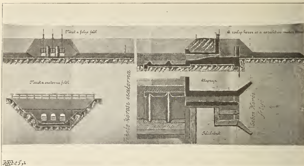
ÖNTÖZŐ-CSATORNA ÉS TÁPLÁLÓ ZSILIP A SEBES-KÖRÖSÖN.
