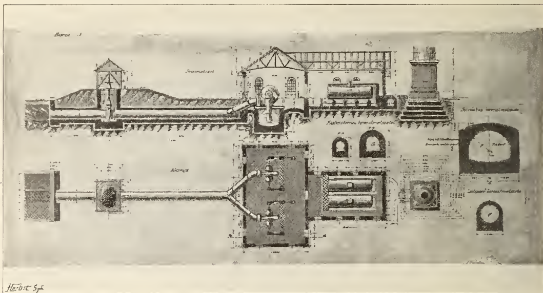
A BORZI SZIVATTYÚTELEP.
