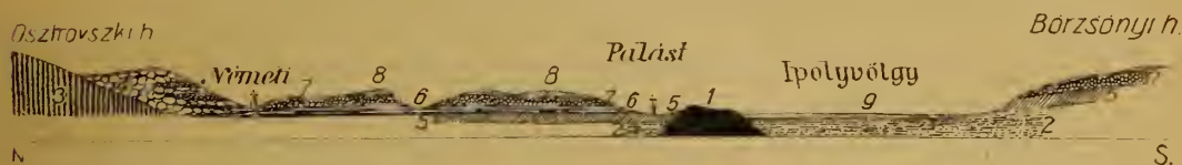
3. ábra. Az Ipoly völgyének vázlatos szelvénye. 1. Grauwacke; 2. mediterrán homok; 3. trachit; 4. trachit breccsa és konglomerát; 5. tömött tufa; 6. homokos tufa; 7. trachit konglomerát; 8. lősz; 9. alluvium; (Sóbányi nyomán).
