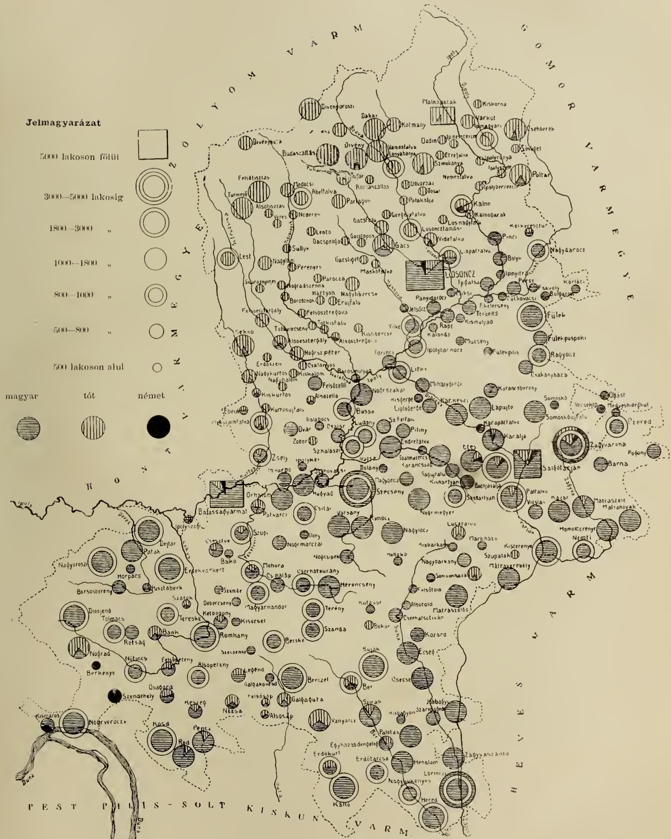
Nógrád vármegye nemzetiségi és népsűrűségi térképe.
