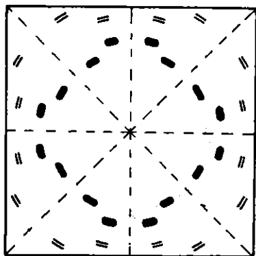
A sugarak elhajlása négytagu szimmetria szerint.
