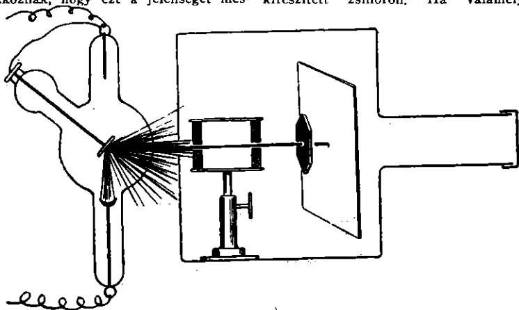
Készülék a Röntgen-sugarakkal való fotografáláshoz.
