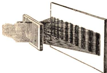
A rácson átbocsájtott fénysugarak elhajlása.
