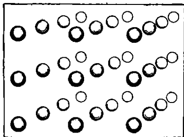
A molekulák elhelyezkedése egy kristályos tér-rácban.
