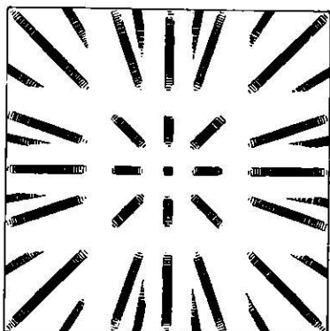
A kereszt-rácson átbocsájtott sugarak elhajlási képe.
