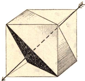
A hármasszimmetriájú lemez helyzete a kockában.
