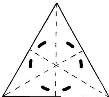
A sugarak elhajlása a háromtaguszimmetria szerint.
