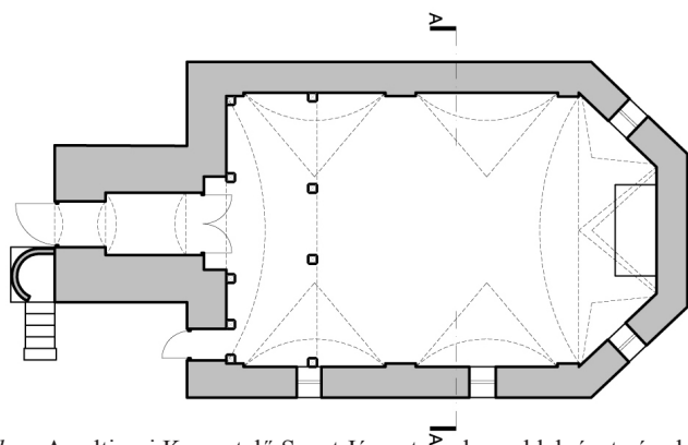
12. ábra. Az altizesi Keresztelő Szent János templom oldalnézete és alaprajza. (Stasisin Izolda felmérése és rajza, 2005)
