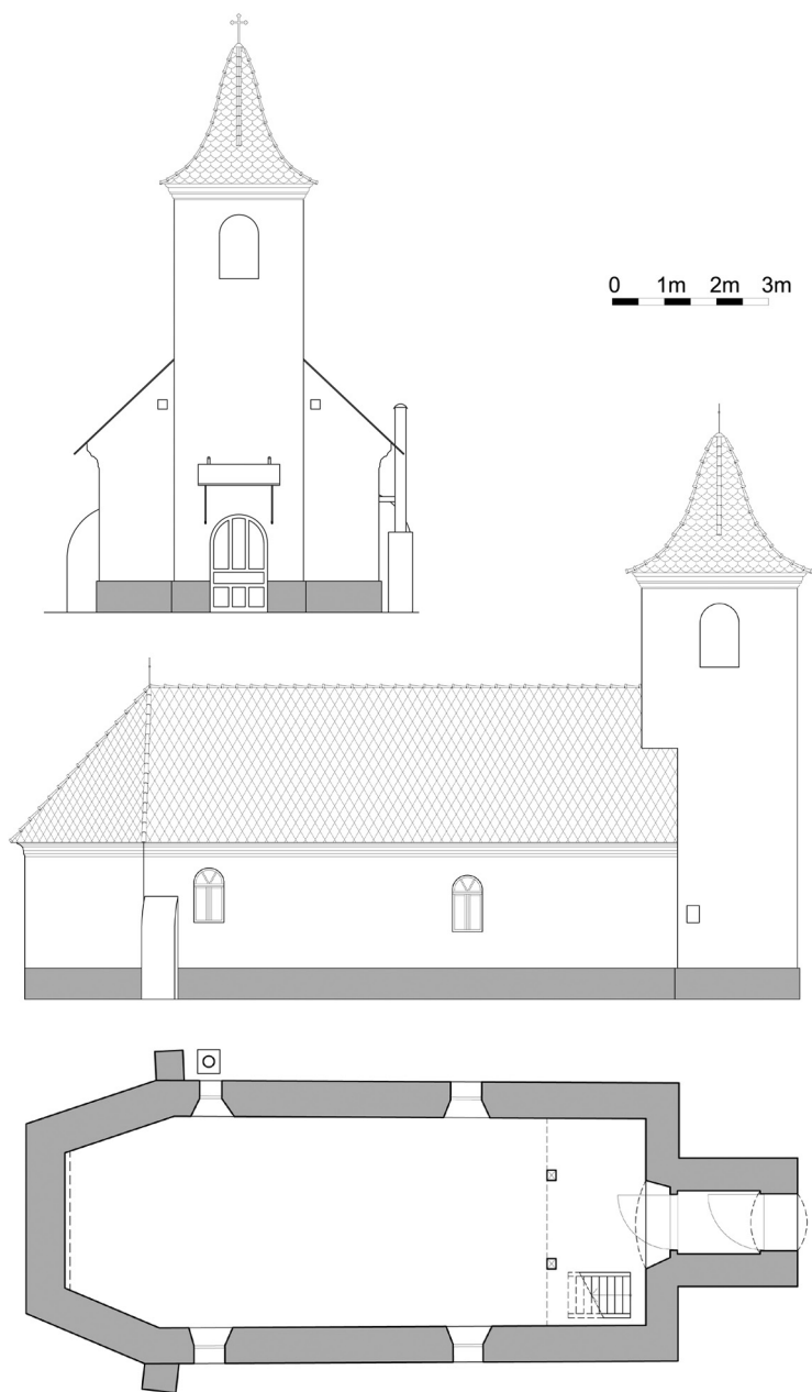
17. ábra. A kötormányi Sarlós Boldogasszony templom előlnézete, oldalnézete és alaprajza. (Stasisin Izolda felmérése, 2005)
