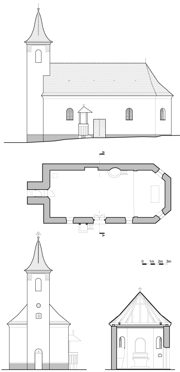
15. ábra A „kálváriai” Jézus szenvedése templom oldalnézete, alaprajza, előlnézete és szentélyének metszete. (Stasisin Izolda felmérése, 2005)
