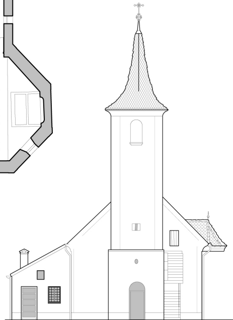
16. ábra. A háromtizesi Szent Kereszt templom oldalnézete, alaprajza, előlnézete. (Stasisin Izolda felmérése, 2005)
