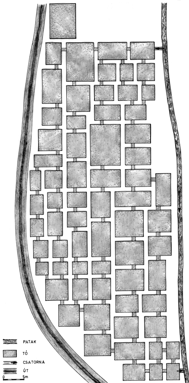
11. ábra. A háromtizesi kenderáztató tók hajdani működtetésének rekonstrukciója. (Tervezte: Bárbth János)
