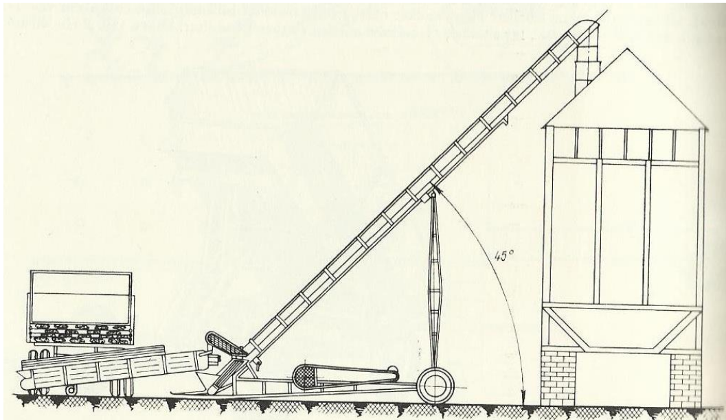
6. ábra. „Vízszintes etető-adagoló szerkezettel ellátott szovjet gyártmányú univerzális felhordó.”
